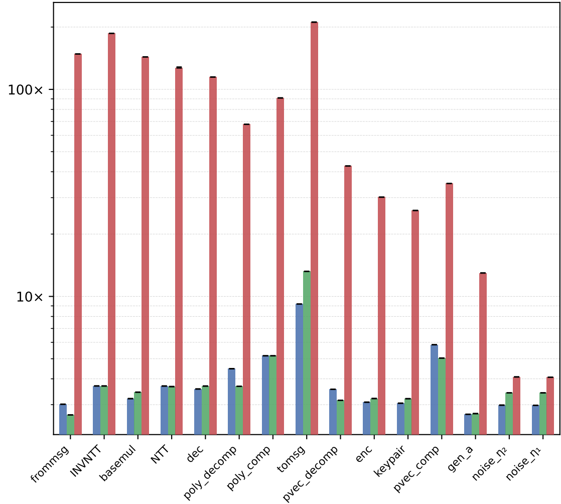
ML-KEM-1024
