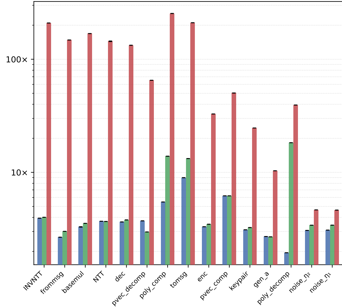
ML-KEM-768
