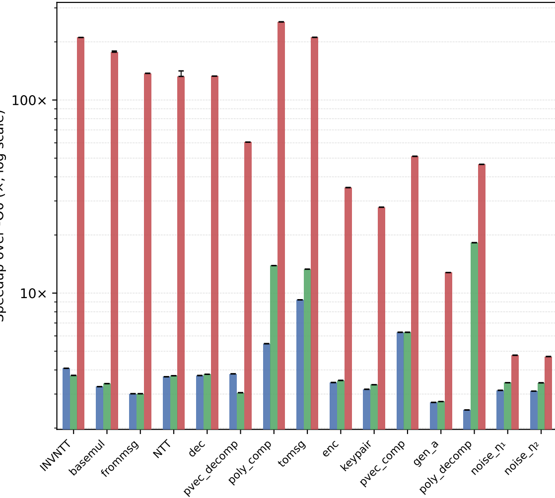
ML-KEM-512
